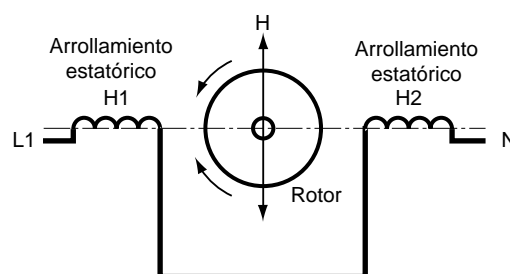
Fig. 9: Principio de funcionamiento de un motor asíncrono monofásico.
